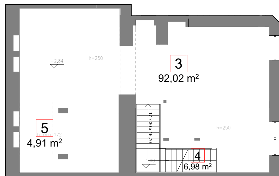
RZUT PIWNICY
