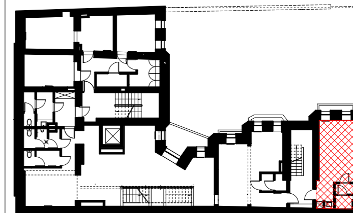
SCHEMAT PIWNICY
