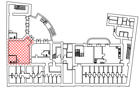
SCHEMAT PIWNICY
